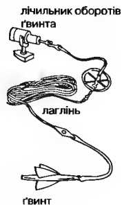
Механічний лаг
